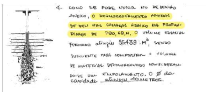
Figura 29 – Trecho manuscrito acompanhado de desenho esquemático da Mina 3, destacados da página 22 (fls. 818 dos autos), do documento 2, da Tabela 1, evidenciando o desmoronamento da cavidade e colapso do topo adentrando nas unidades geológicas sotopostas à camada de sal.
