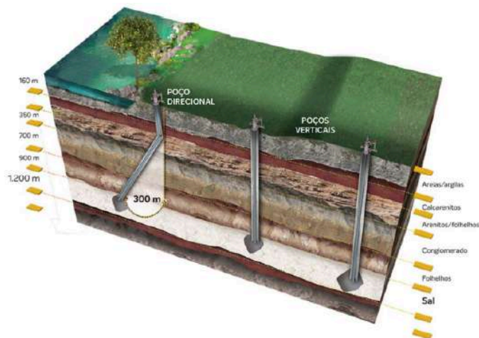
Figura 3 – Tipos de poços na extração de sal-gema e camadas geológicas atravessadas - Fonte: https://www.braskem.com.br/detalhe-noticias-de-alagoas/extracao-em-infograficos .
