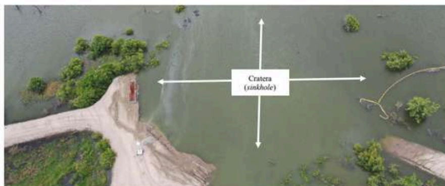
Figura 57 – Cratera ( sinkhole ) de aproximadamente 150 metros de diâmetro formada na região da Mina 18D em 10/12/2023, em imagem aérea registrada pela Perícia em 11/12/2023.
