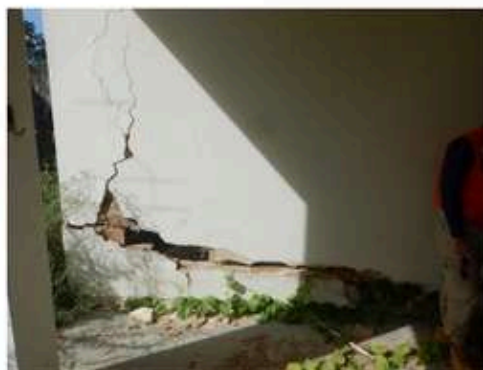
Figura 49 – Aberturas generalizadas e deslocamento em painéis de habitação residencial térrea.
