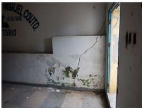
Figura 52 – Aberturas diagonais em painéis e recalques no piso em edificação com dois pavimentos.
