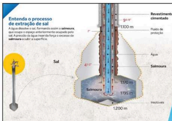
Figura 7 - Representação de um poço vertical de sal-gema com injeção de água pelo tubo central e extração de salmoura pelo espaço anular adjacente
